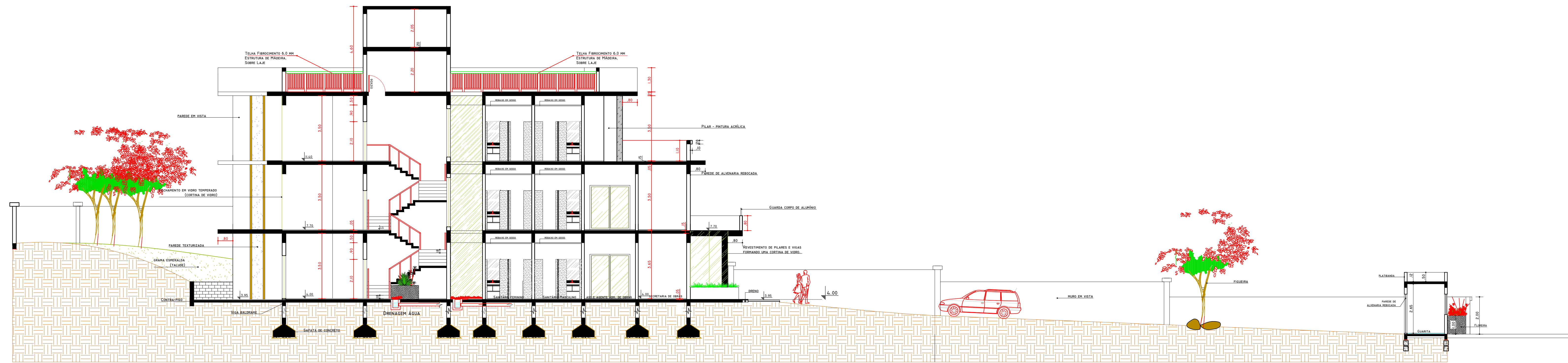
CORTE LONGITUDINAL AA'
